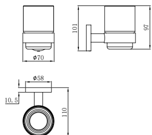
Portavaso y vaso de pared • Vaso de vidrio • Soporte metálico • Instalación mural
