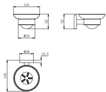
Jabonera con soporte • Jabonera de vidrio • Soporte metálico • Instalación mural
