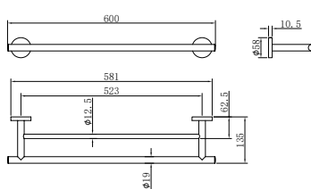
Toallero doble • 60 cm • Metálico • Instalación mural
