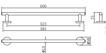
Toallero • 30 cm (ref. 170900200) • 60 cm • Metálico • Instalación mural
