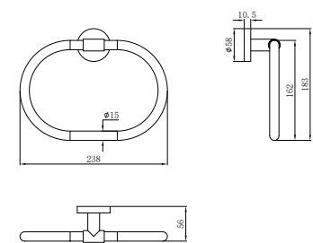
Toallero de anillo • 23,8 cm • Metálico • Instalación mural
