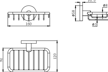
Jabonera con soporte • Metálico • Instalación mural
