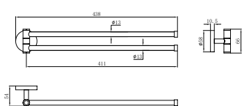
Toallero basculante • 43,8 cm • Metálico • Instalación mural
